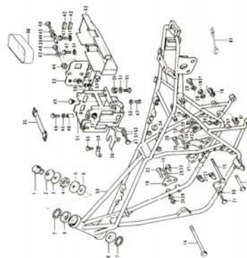
17. Frame 1/2
