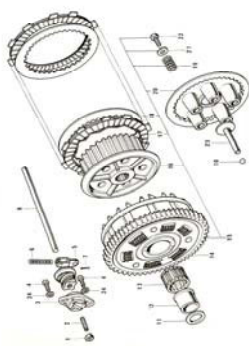
7. Clutch
