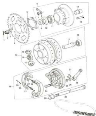
24. Rear Hub
