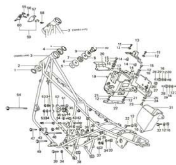
17. Frame 1/2
