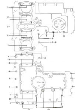
6. Crank Case Bolt & Stud Pattern
