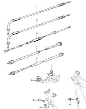
31. Cables
