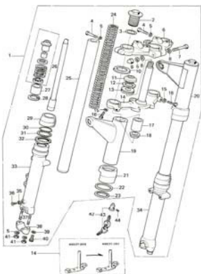
27. Front Fork1/2
