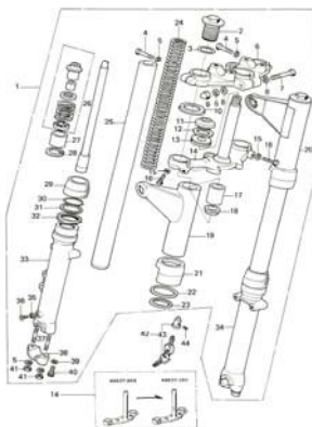
27. Front Fork2/2
